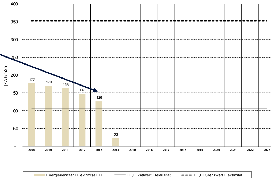
Energiekennzahl Elektrizität E_{\square} nutzungskorrigiert
